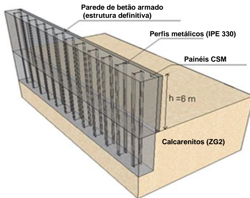
Figura 5 – Esquematização da Solução Adoptada: a) Planta da Escavação e da Área Envolvente; b) Aspecto Tridimensional da Solução Estrutural Adoptada
